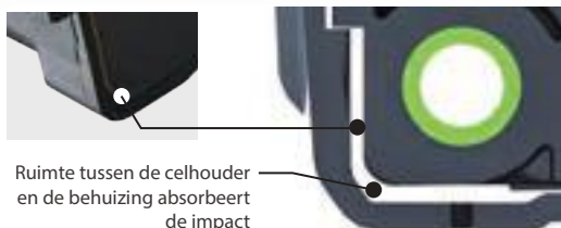
Schokabsorberende structuur
