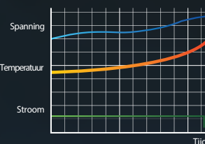
Standaard laadtraject
